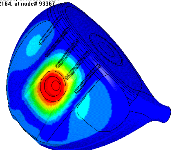
模態振動模擬
